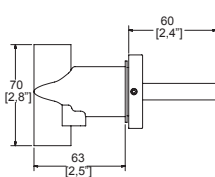
Dimensión lateral:
