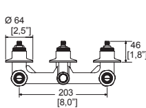
Dimensión cenital:
