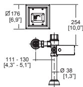
Dimensión frontal:
