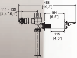
Dimensión lateral:
