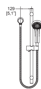
Dimensión lateral:
