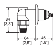
Dimensión lateral:
