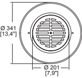
Dimensión cenital:
