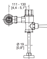
Dimensión frontal:
