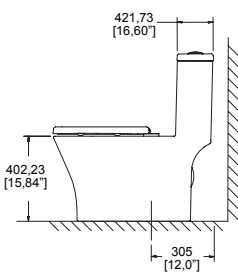
Dimensión lateral:
