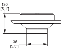
Dimensión lateral:
