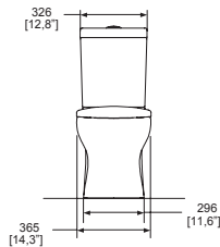
Dimensión frontal:
