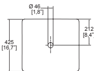
Dimensión cenital:
