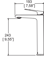
Dimensión lateral:
