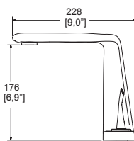
Dimensión lateral:
