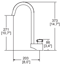
Dimensión lateral:
