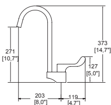
Dimensión lateral:
