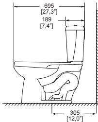
Dimensión lateral:
