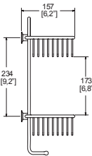
Dimensión lateral:
