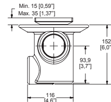
Dimensión lateral:
