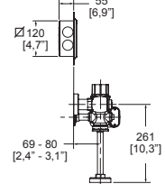
Dimensión lateral:
