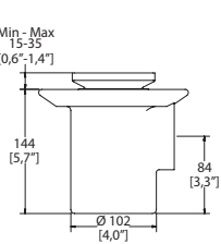
Dimensión lateral:
