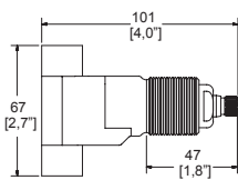
Dimensión lateral:
