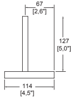
Dimensión lateral:
