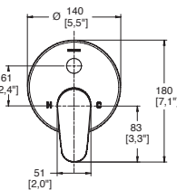
Dimensión frontal:
