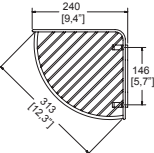
Dimensión lateral:
