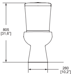
Dimensión frontal:
