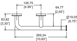
Dimensión cenital:
