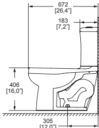
Dimensión lateral:
