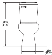
Dimensión frontal:
