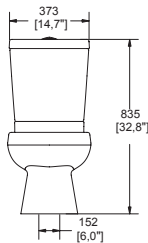
Dimensión frontal:
