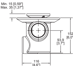
Dimensión lateral:
