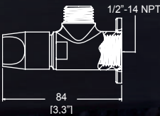
Dimensión lateral:
