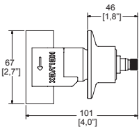
Dimensión lateral:
