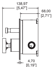
Dimensión lateral:
