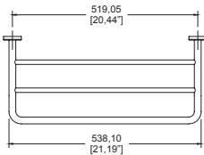
Dimensión cenital:
