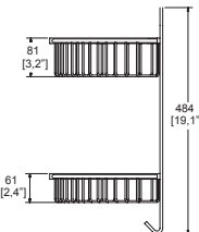
Dimensión lateral:
