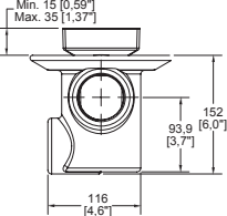
Dimensión lateral:
