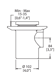
Dimensión lateral:
