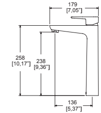
Dimensión lateral:
