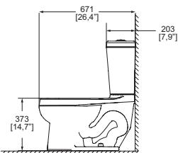
Dimensión lateral:
