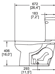
Dimensión lateral:
