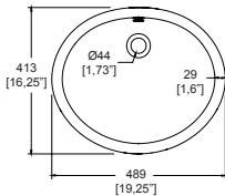
Dimensión cenital:
