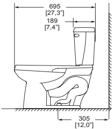
Dimensión lateral:
