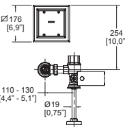
Dimensión frontal:
