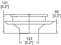
Dimensión frontal:
