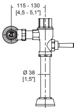
Dimensión frontal:
