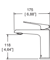
Dimensión lateral:
