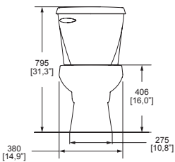
Dimensión frontal:
