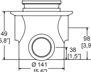
Dimensión lateral:
