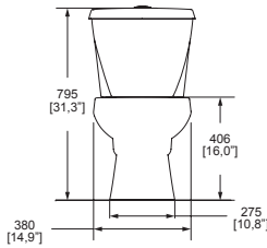
Dimensión frontal:
