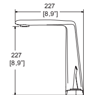
Dimensión lateral:
