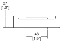
Dimensión frontal:
