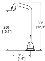
Dimensión lateral:
