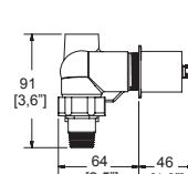
Dimensión lateral:
